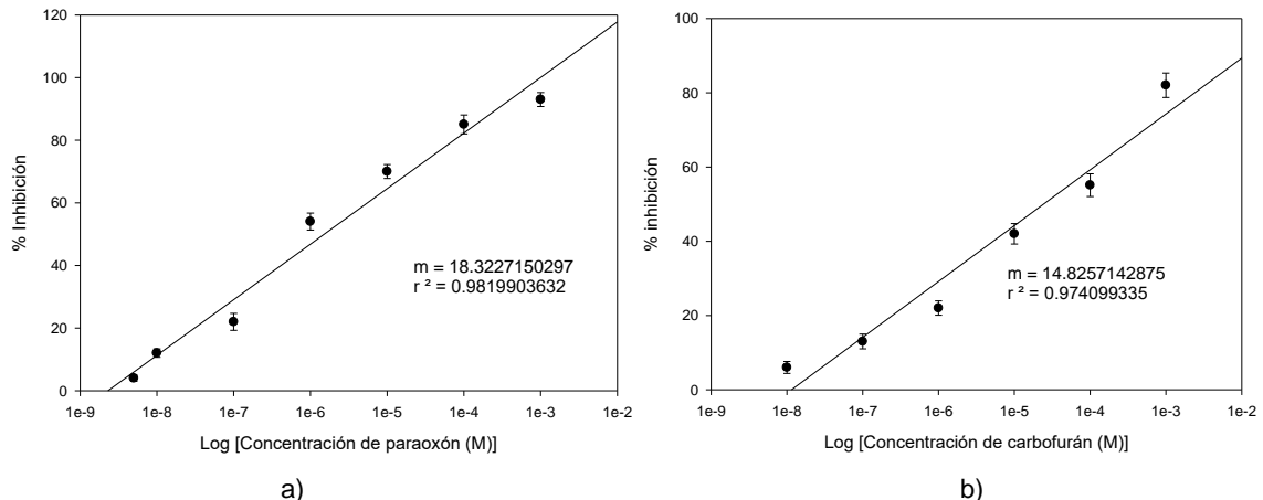
Figura 11. Porcentaje de Inhibición en la respuesta del EnFET respecto del a) Paraoxón y b) Carbofurán.
