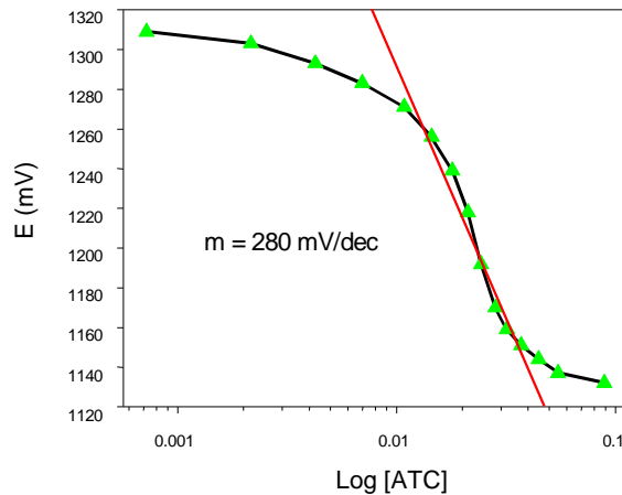
Figura 10. Gráfica de potencial del EnFET respecto de la concentración de acetilcolina.
