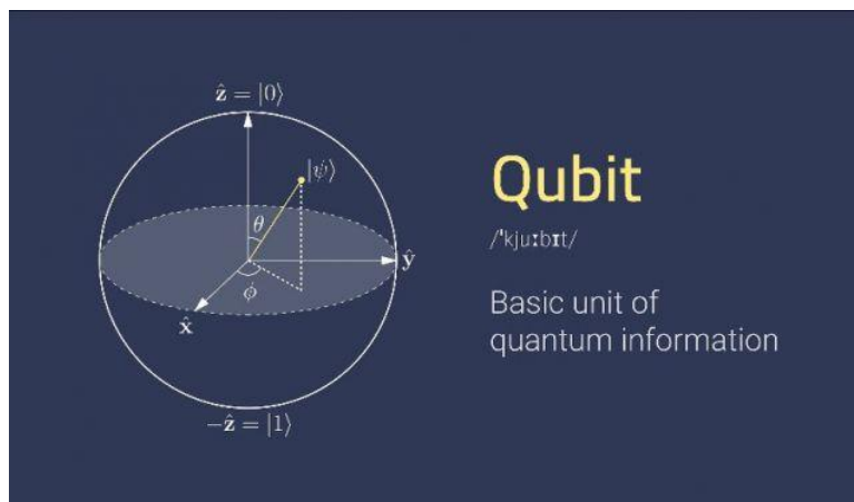
Figura 1. Bit cuántico.
