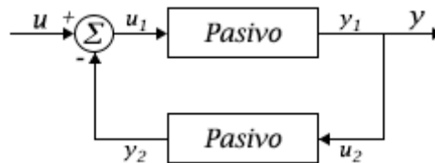
Figura 2. Sistemas pasivos interconectados.
